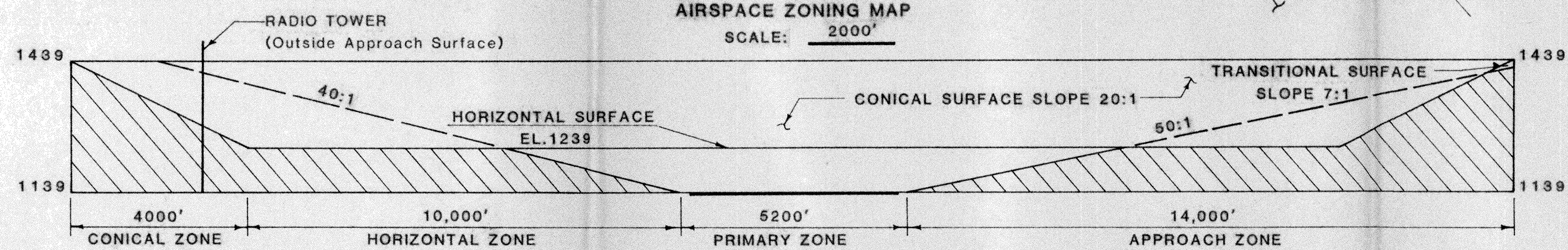
SECTION A-A
